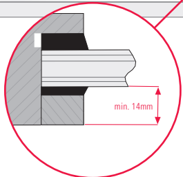
Detail: rechtwinkelige Glasleiste
