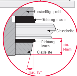
Detail: schräge Glasleiste
