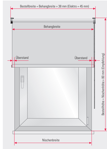
freihängend Wandmontage
