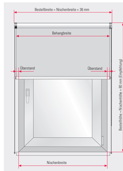
Seitenzug oder Elektro mit Spanndraht- führung Wandmontage
