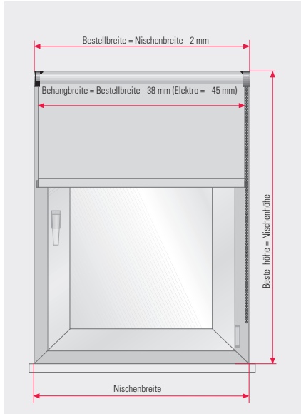
freihängend Nischenmontage
