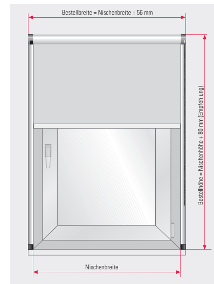
Seitenzug oder Elektro mit SunTape- Seitenführung Wandmontage
